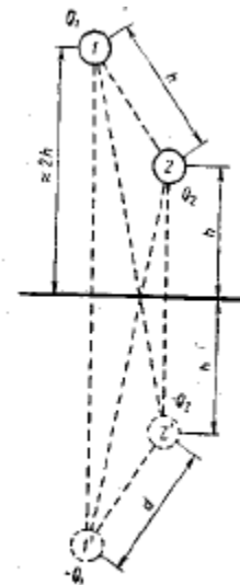
Рис. 13. Схема расположения проводов линии электропередачи
